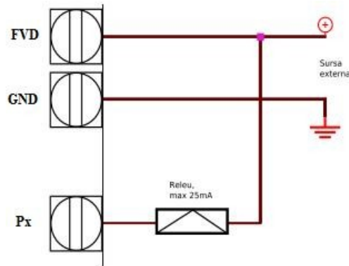
Fig. 3 - diagramă conectare port ieşire modul
